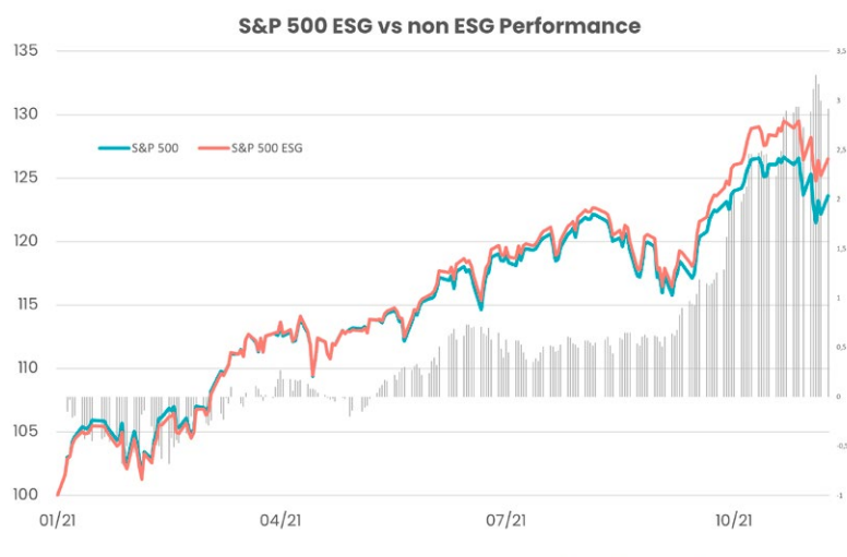
Graf porovnania vývoja amerických akciových indexov S&P 500 a S&P 500 ESG
